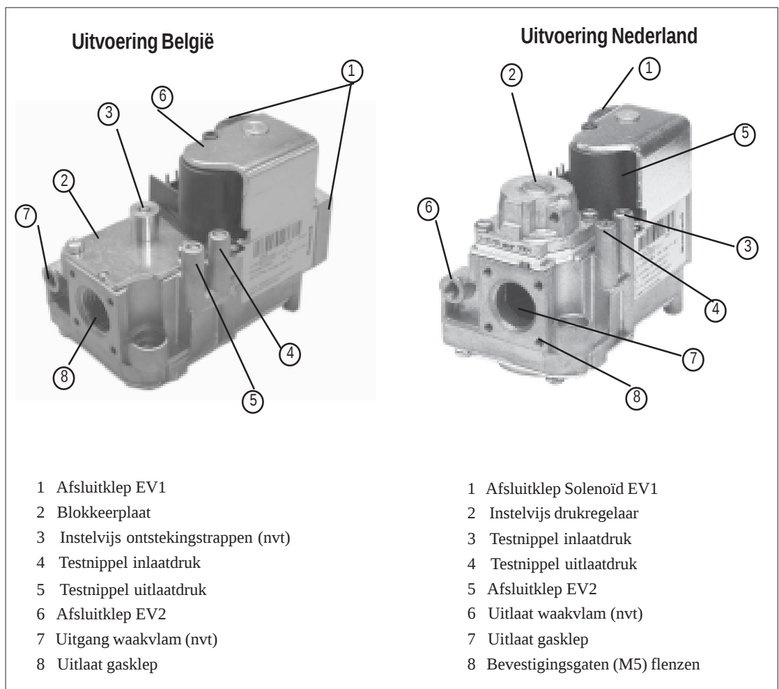
Figuur 10a : Honeywell gasklep types 008-2 -> 030-2
