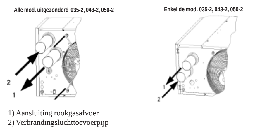
Figuur 5 : Type C-installatie : Aansluitingen luchttoevoer & rookgasafvoer
