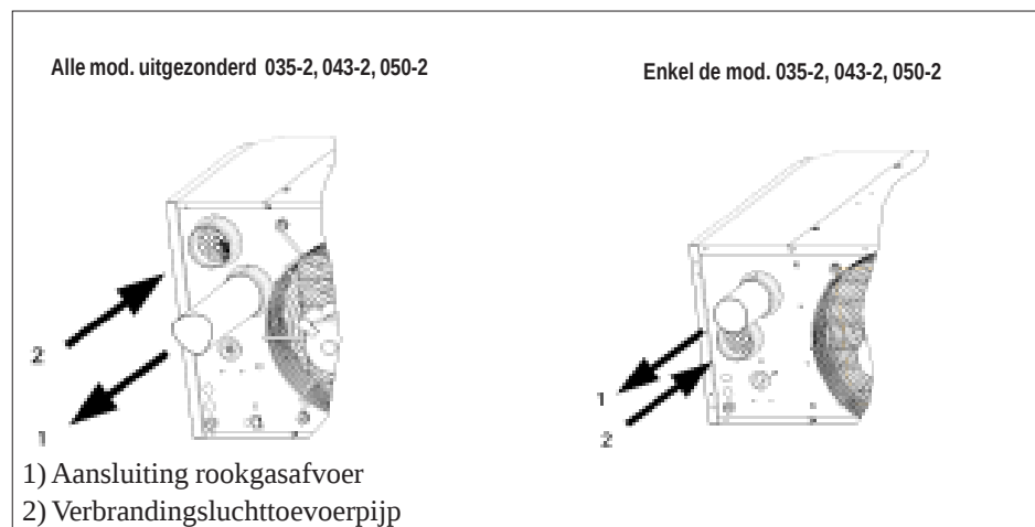
Figuur 3 : Type B installatie : Aansluitingen luchttoevoer & rookgasafvoer
