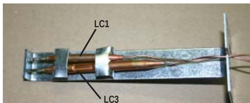
Figuur 25 : LC1/LC3 plaatsaanwijzing
