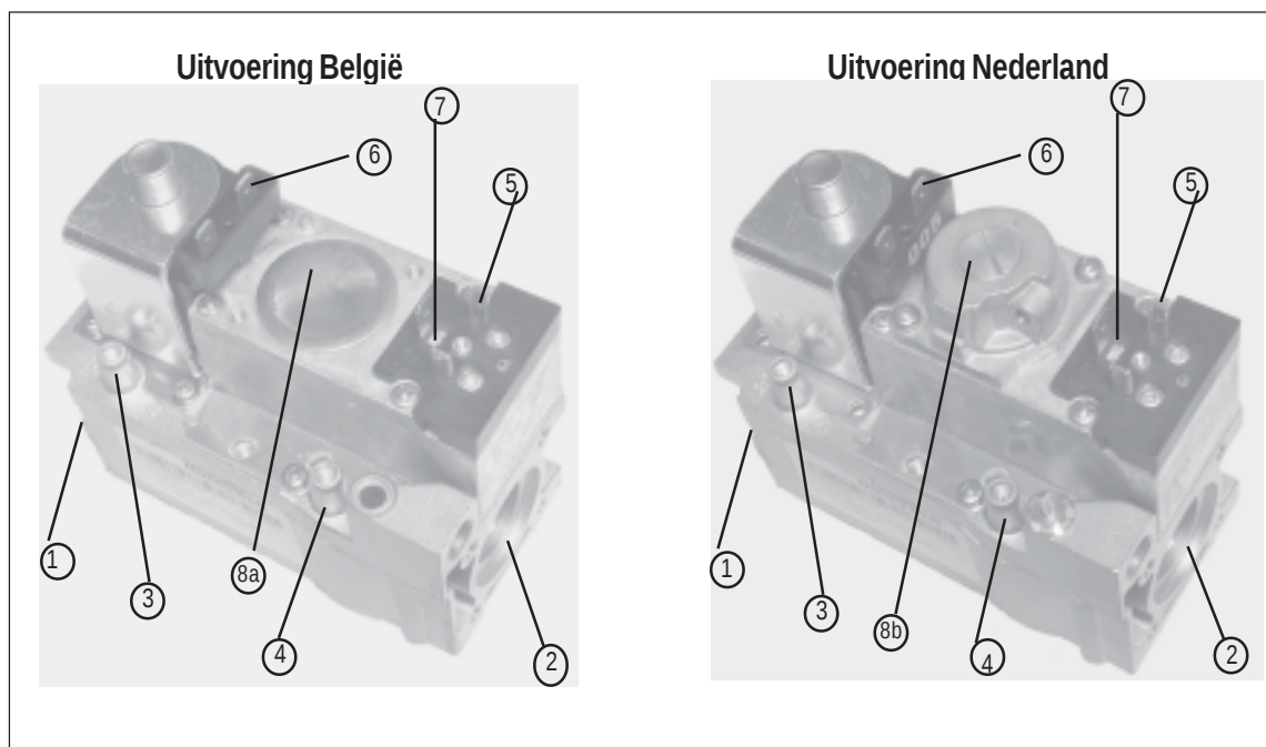
Figuur 10b : Honeywell gasklep type 035-2 -> 100-2
